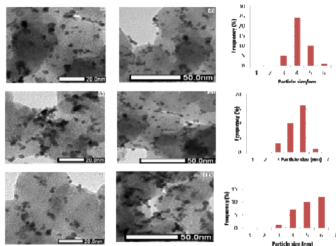
Fig.2:TEM image of nanoparticles catalysts: a),d) PtRuMo/C(3:1:1), b),e) PtRuMo/C(2:1:1), c),f) PtRuMo/C (3:2:1)
